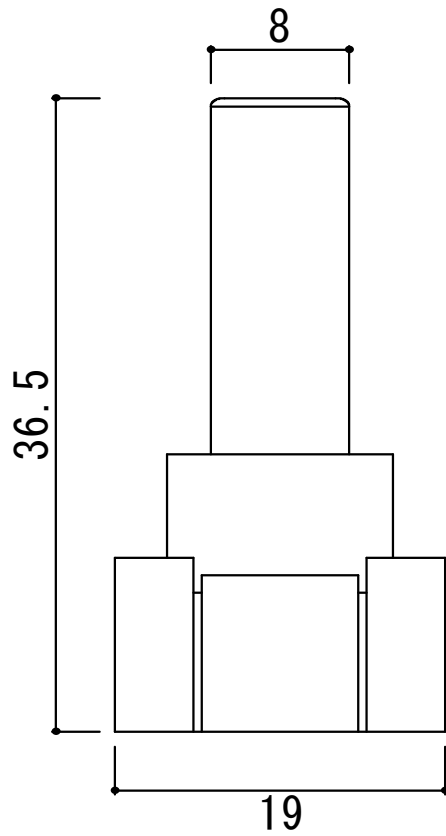
正面图
