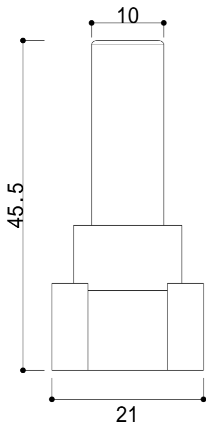
正面图
