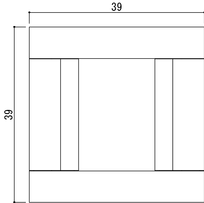
平面图
