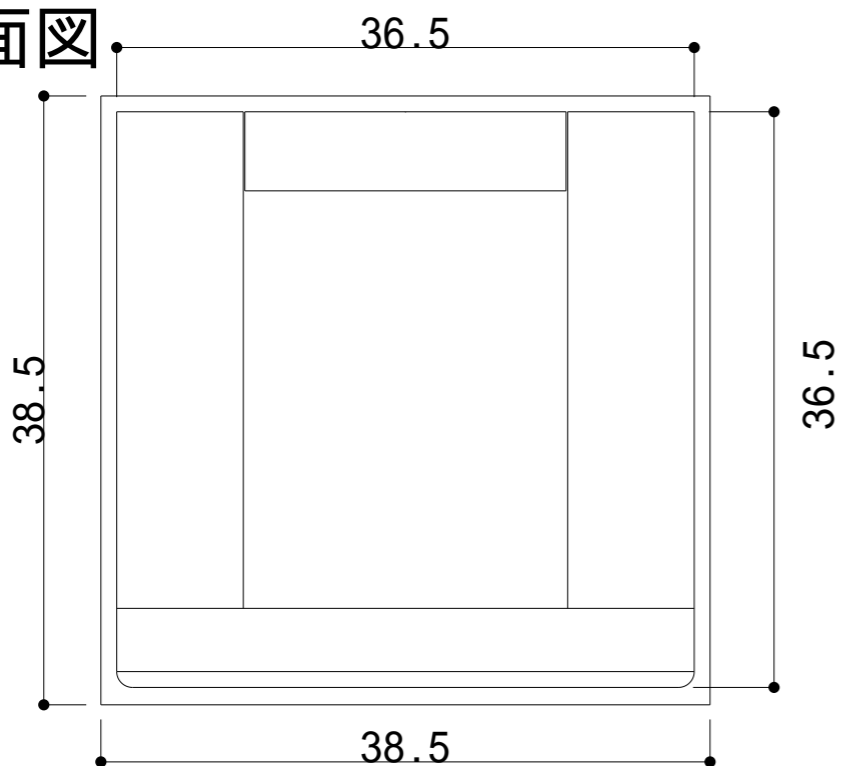
正面圖
