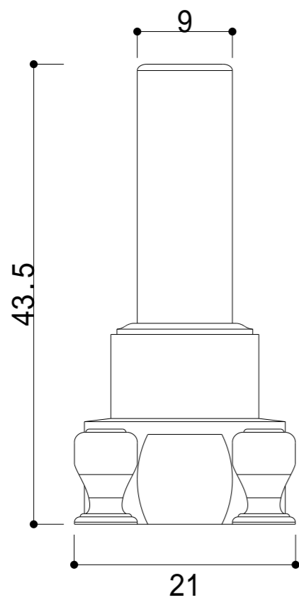
正面圖
