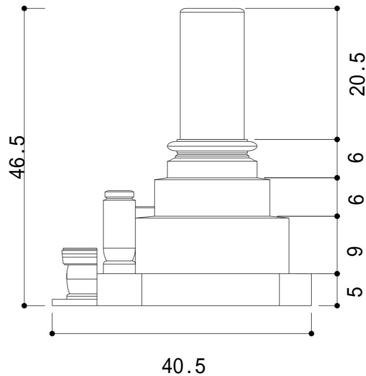
側面圖
