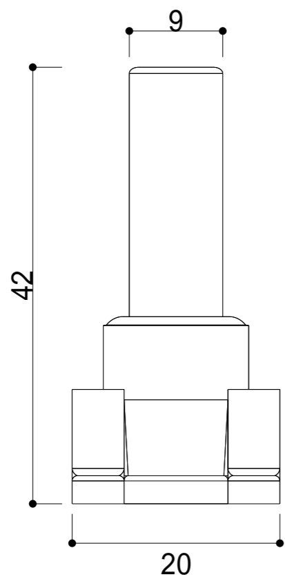
正面圖
