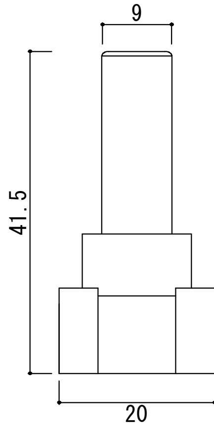
正面圖
