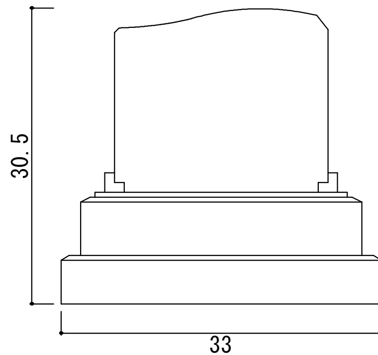
侧面图
