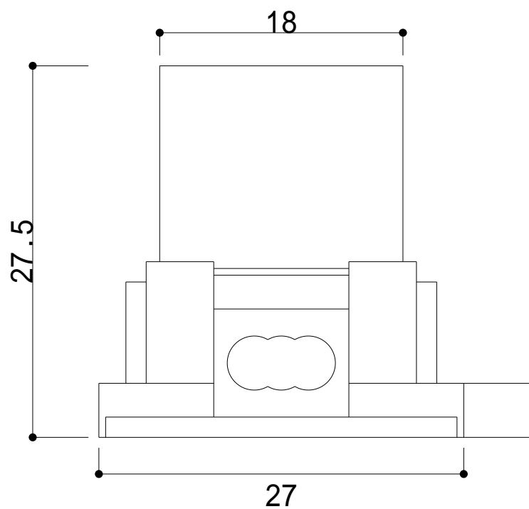
正面圖
