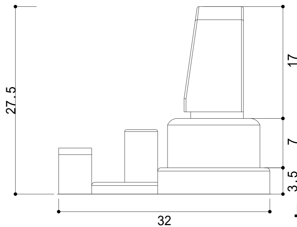
侧面图
