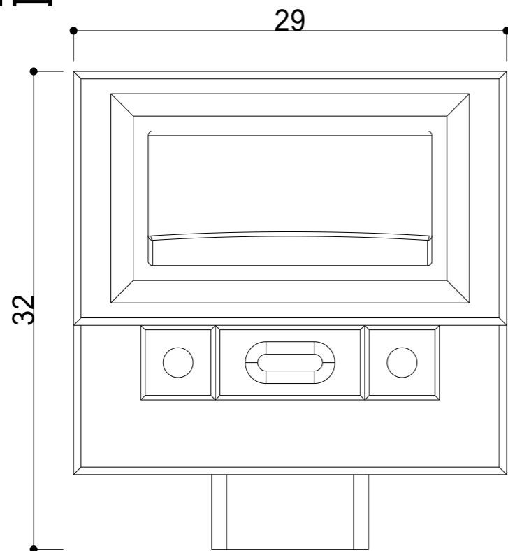
平面图
