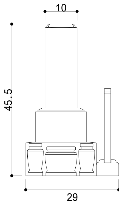
正面图
