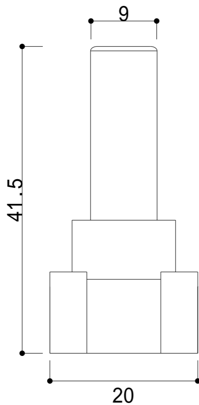
正面图
