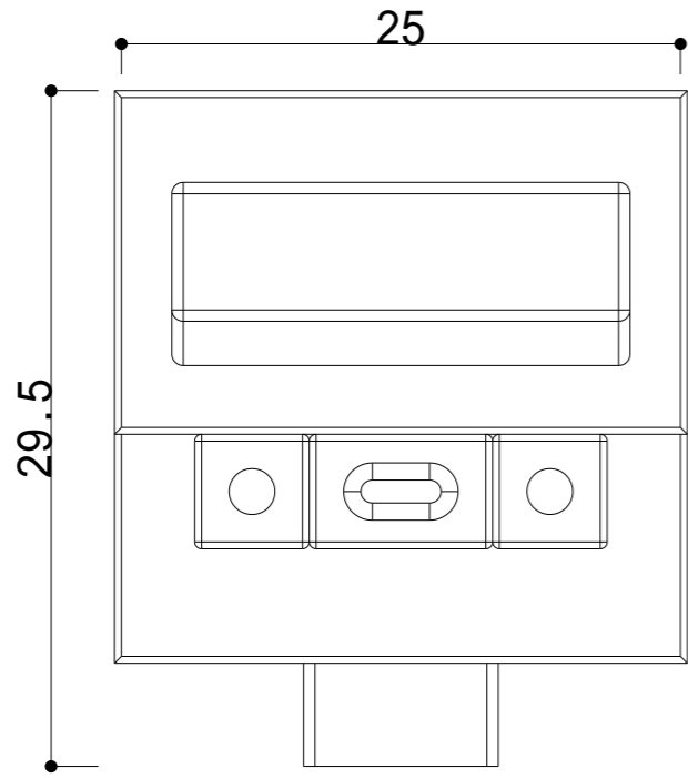
平面圖
