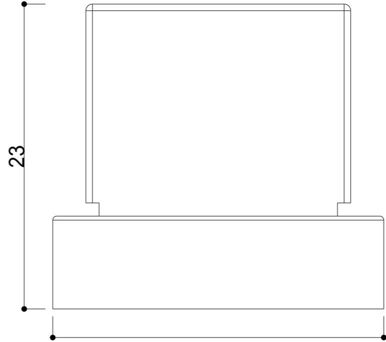
側面圖
