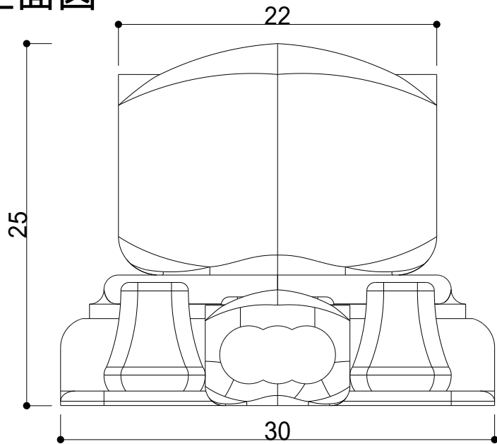
正面圖
