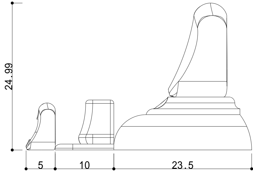
側面圖
