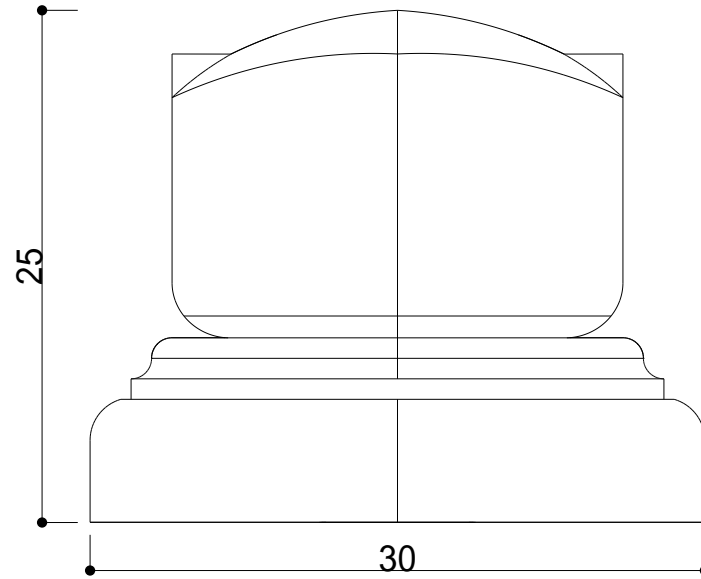
側面圖
