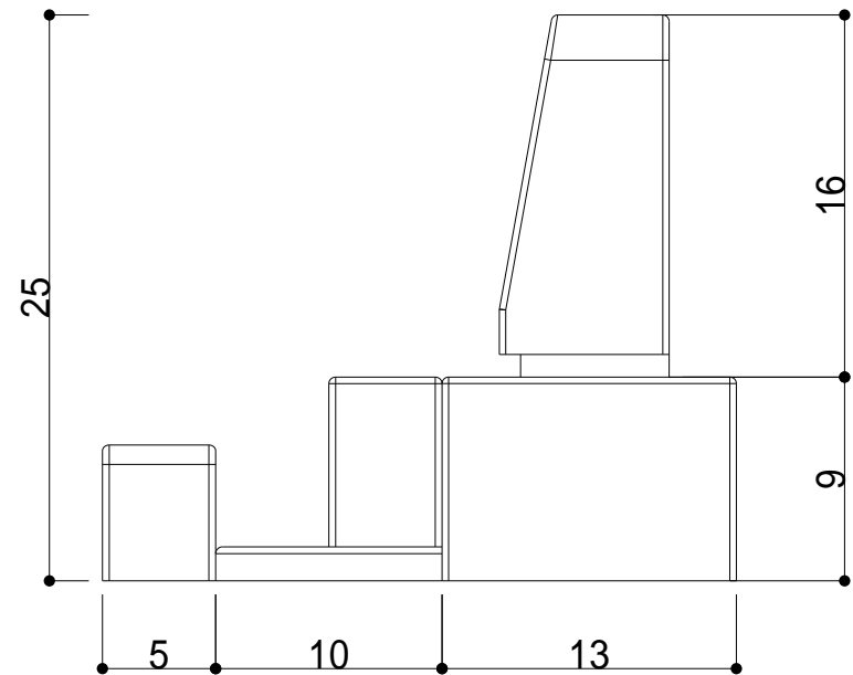
側面圖
