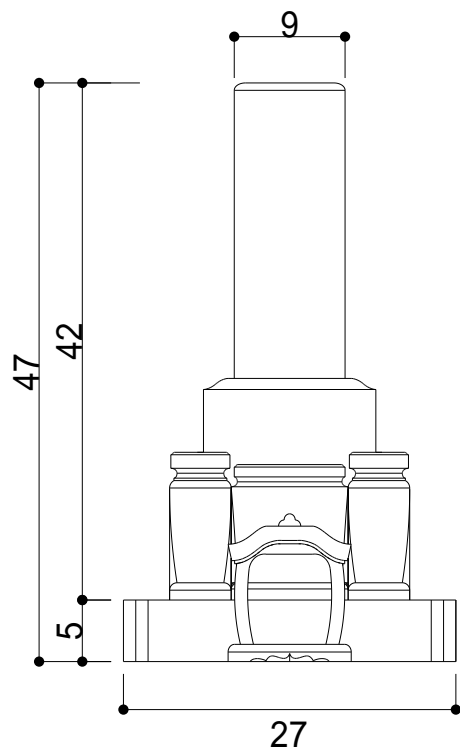
正面圖
