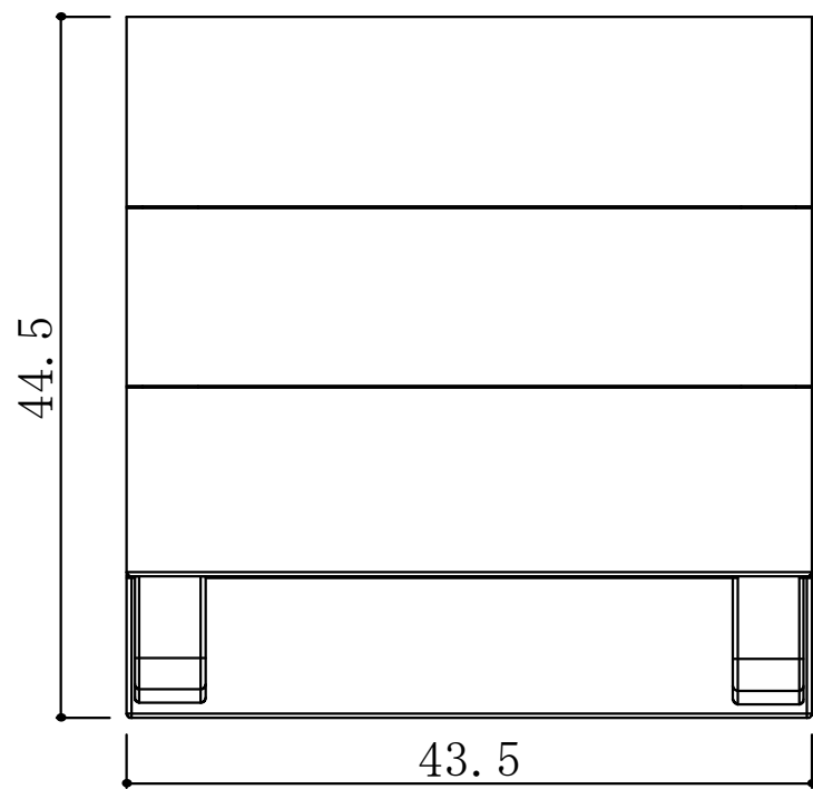
正面圖
