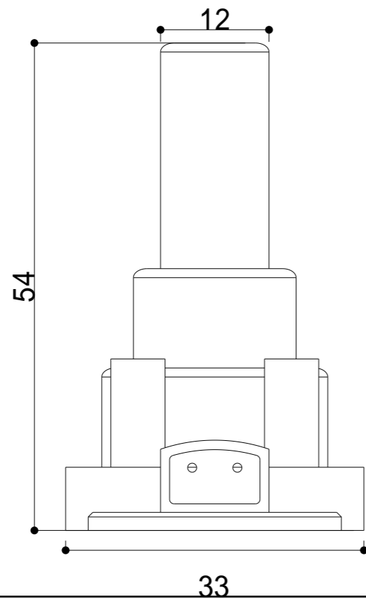
正面圖
