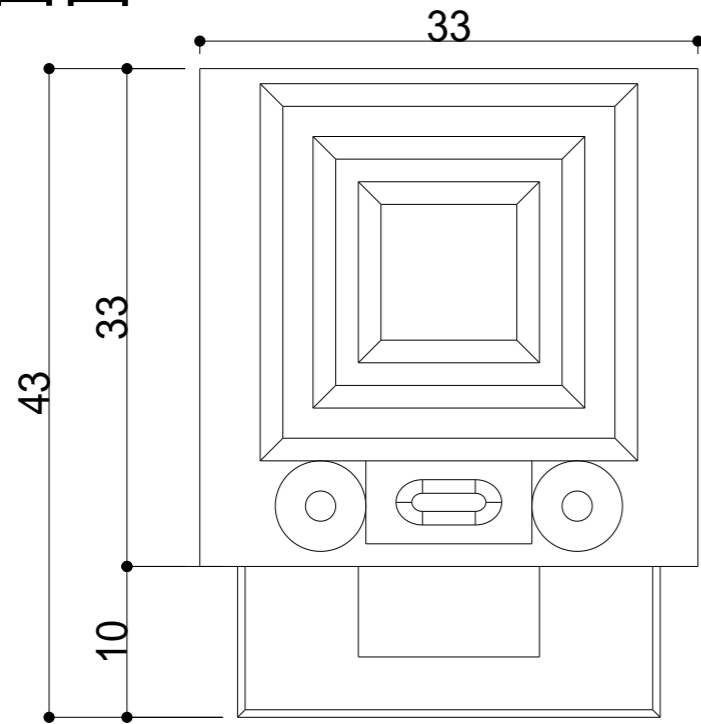
平面圖
