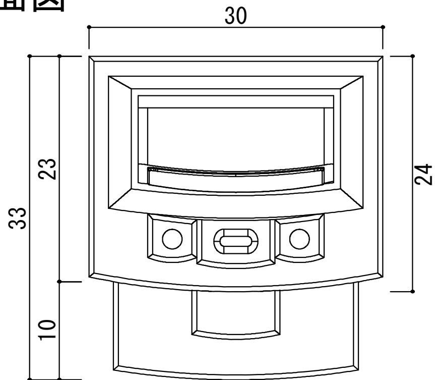
平面圖
