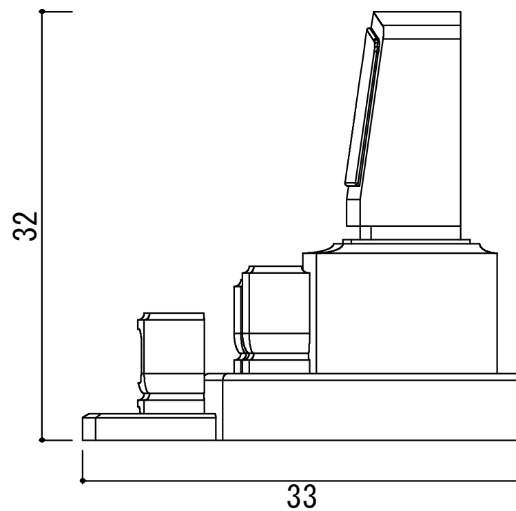
側面圖
