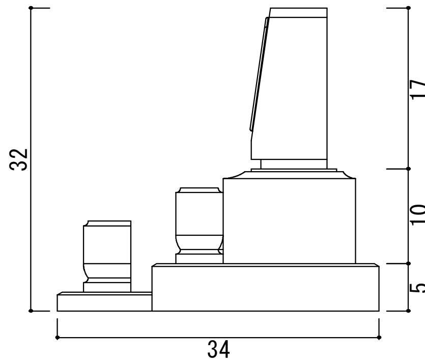
侧面图
