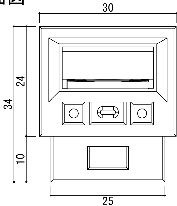
正面图
