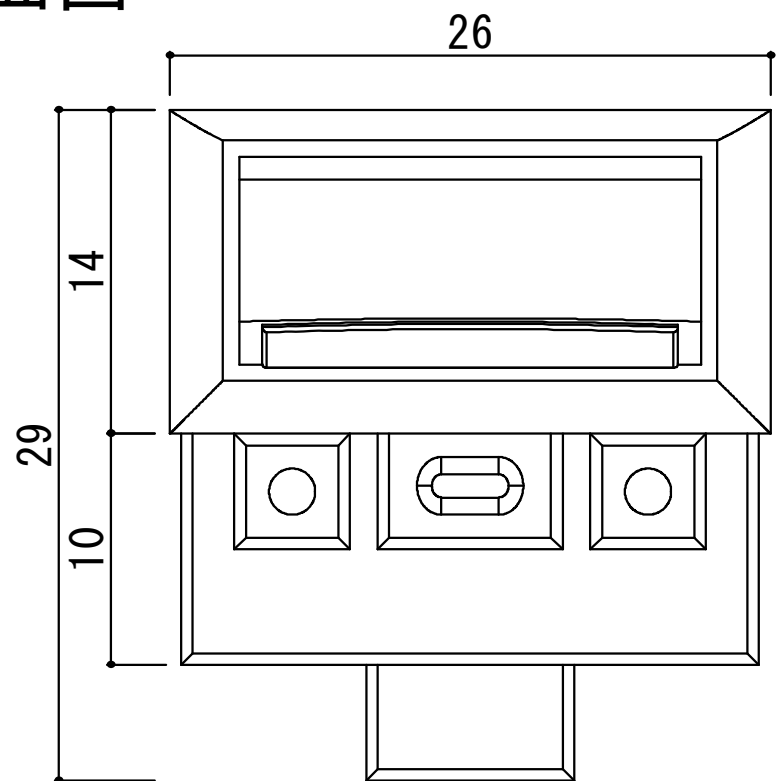
平面圖
