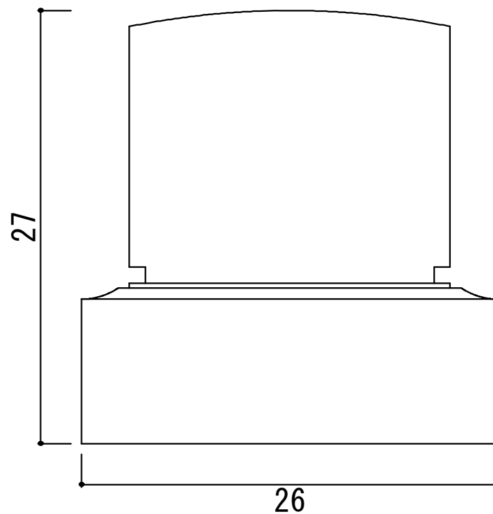
側面圖
