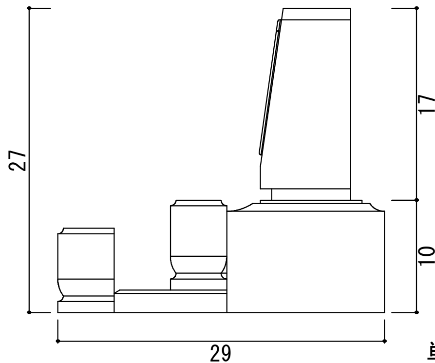
側面圖
