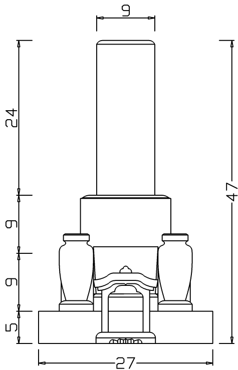
正面图
