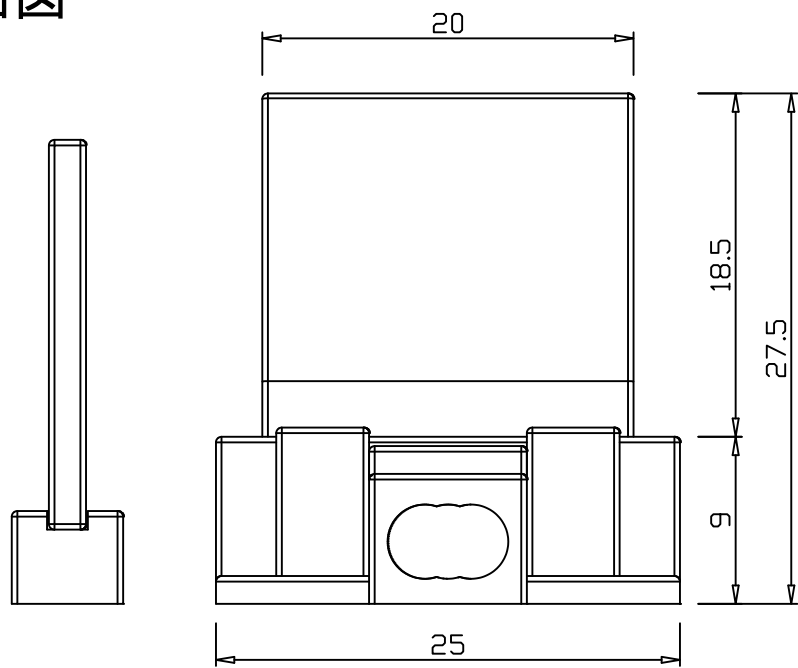
正面図
