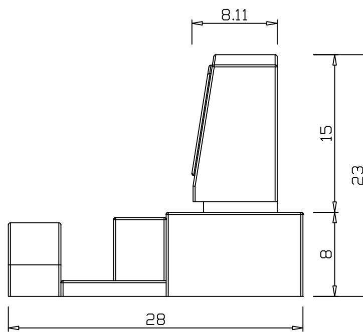
側面図
